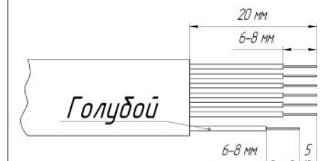
Схема обрезки кабеля
